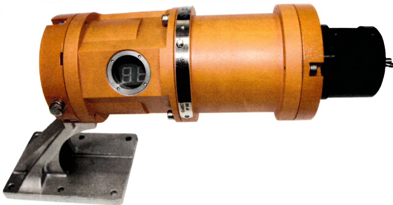
Рисунок 2 - Газоанализаторы СГОЭС-М-2 внешний вид с кронштейном и модулем отображения информации
